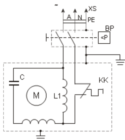
Obrázek A.1 – Schéma elektrických obvodů kompresorů C-50.LB30A, C-100.LB30A, C-100.LB30AB
