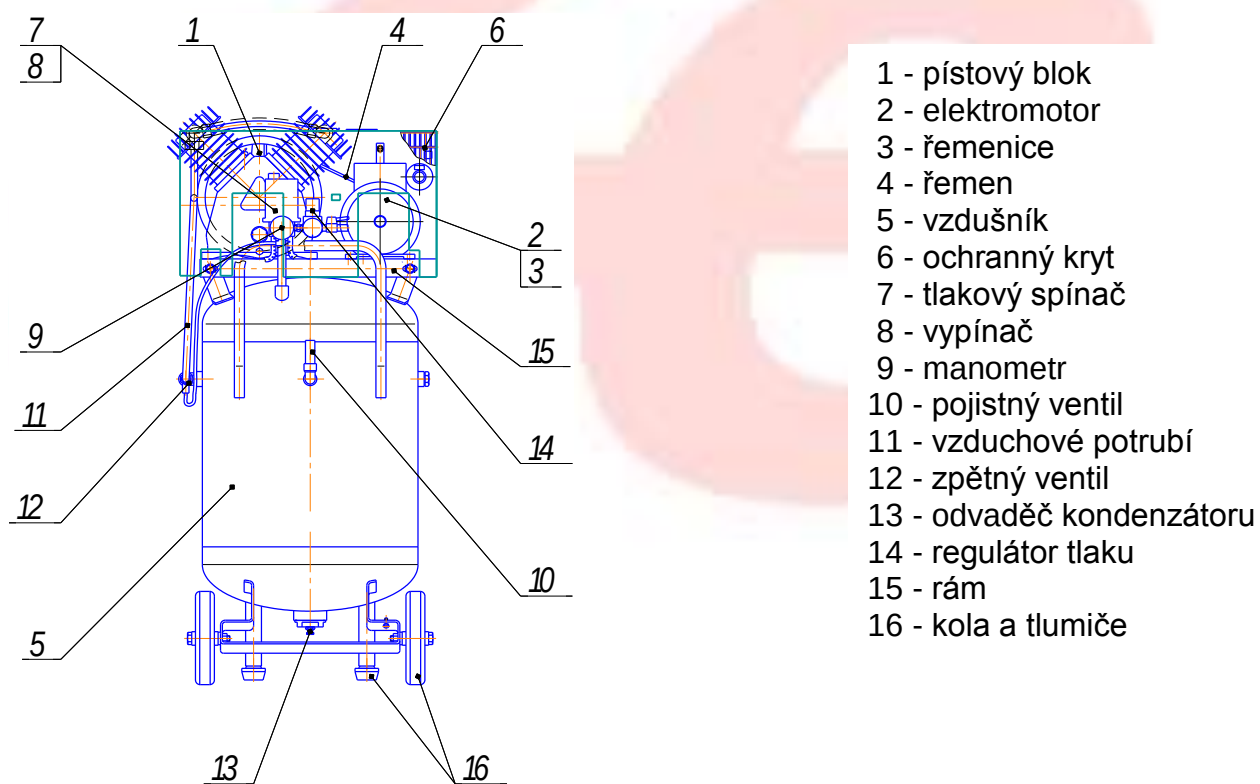
Obr. 7 - Celkový pohled na kompresor C-100.LB30B, C-100.LB30AB
