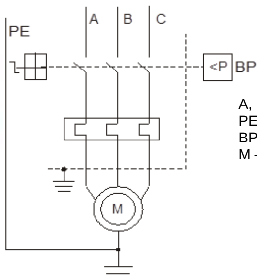
Obrázek A.2 – Schéma elektrických obvodů kompresorů C-50.LB30, C-100.LB30, C-100.LB30B
