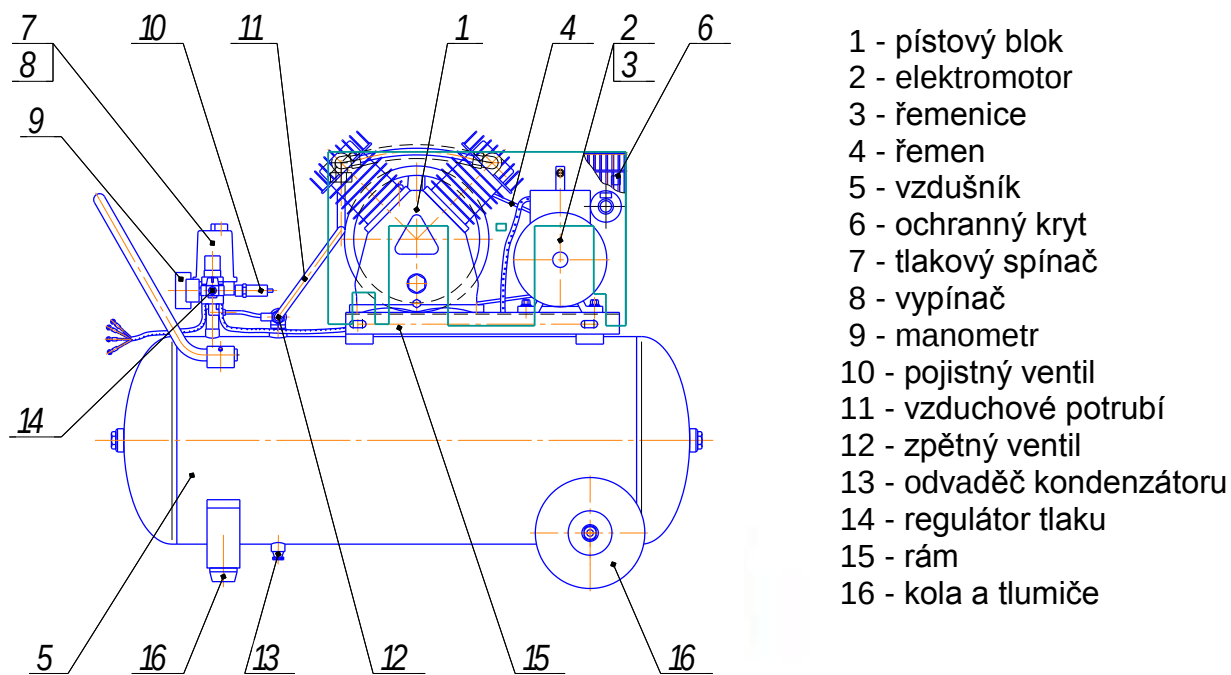
Obr. 6 - Celkový pohled na kompresor C-100.LB30, C-100.LB30A
